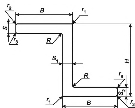
Рисунок 1 — Прессованный прямоугольный профиль равнополочного зетового сечения
