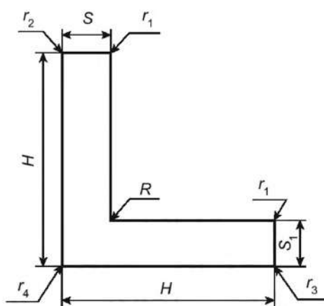
Т а б л и ц а 1 — Норма профилей, размеры и теоретическая масса
