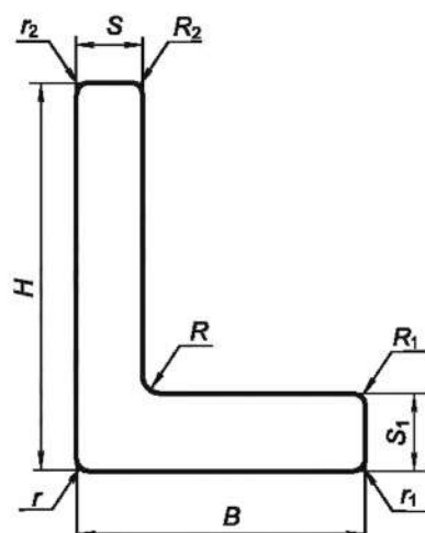
Рисунок 1 — Прессованный прямоугольный профиль неравнополочного углового сечения
