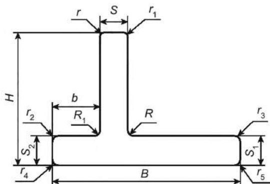
Рисунок 1 — Прессованный прямоугольный профиль неравнополочного таврового сечения
